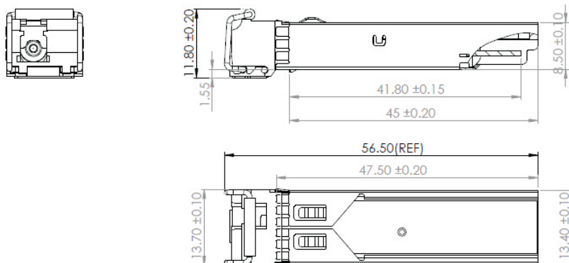
AP5B53303xxL20
